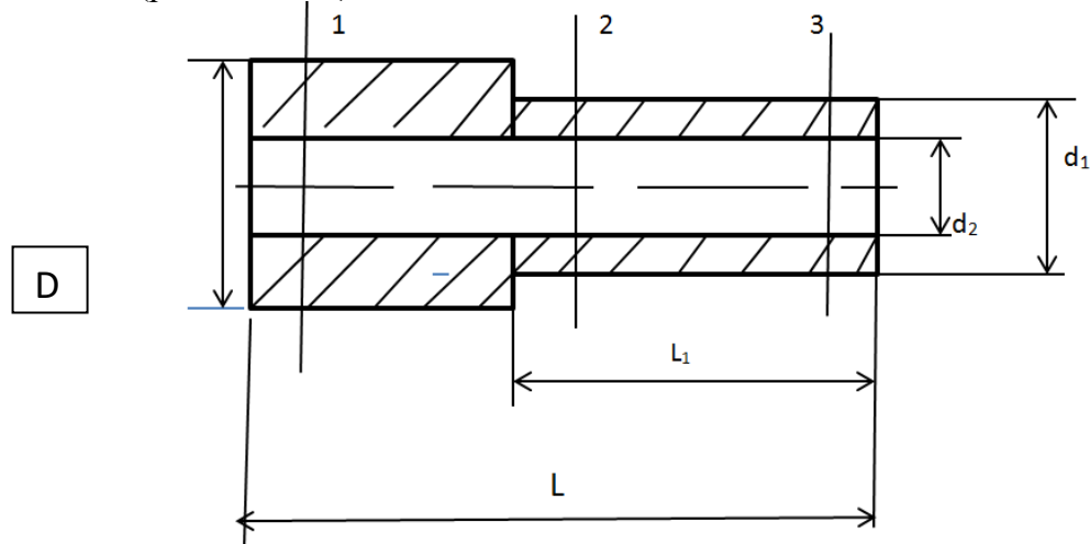
Рисунок 1 Чертеж ступицы
