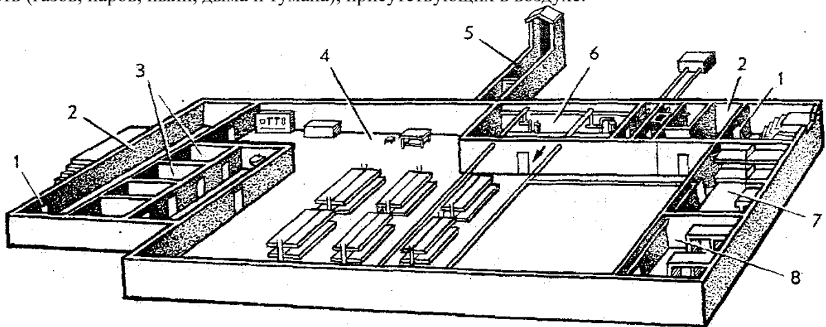
Рисунок 2.1 – План убежища
