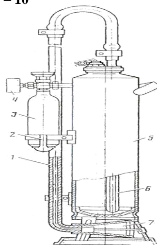
Рисунок 2 - Воздушно-пенный огнетушитель ОВП – 10
