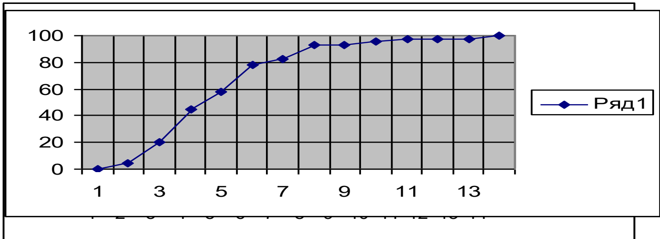
Рисунок 7 – Функция накопленных частот случайной величины D_i для выборки Б.
