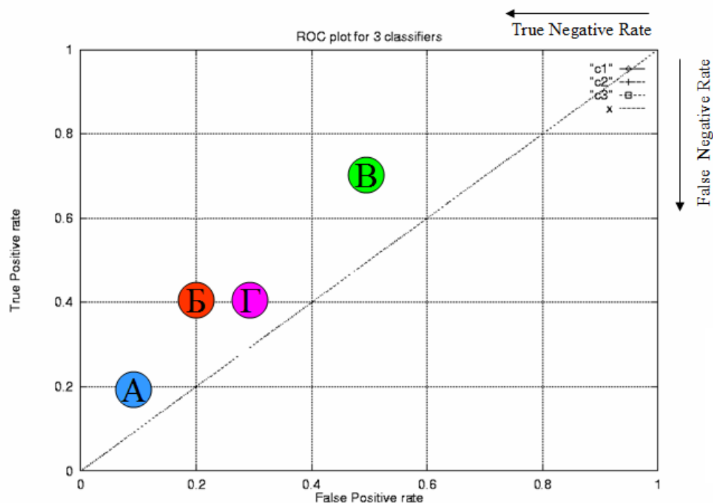
Рис.2. ROC-пространство
