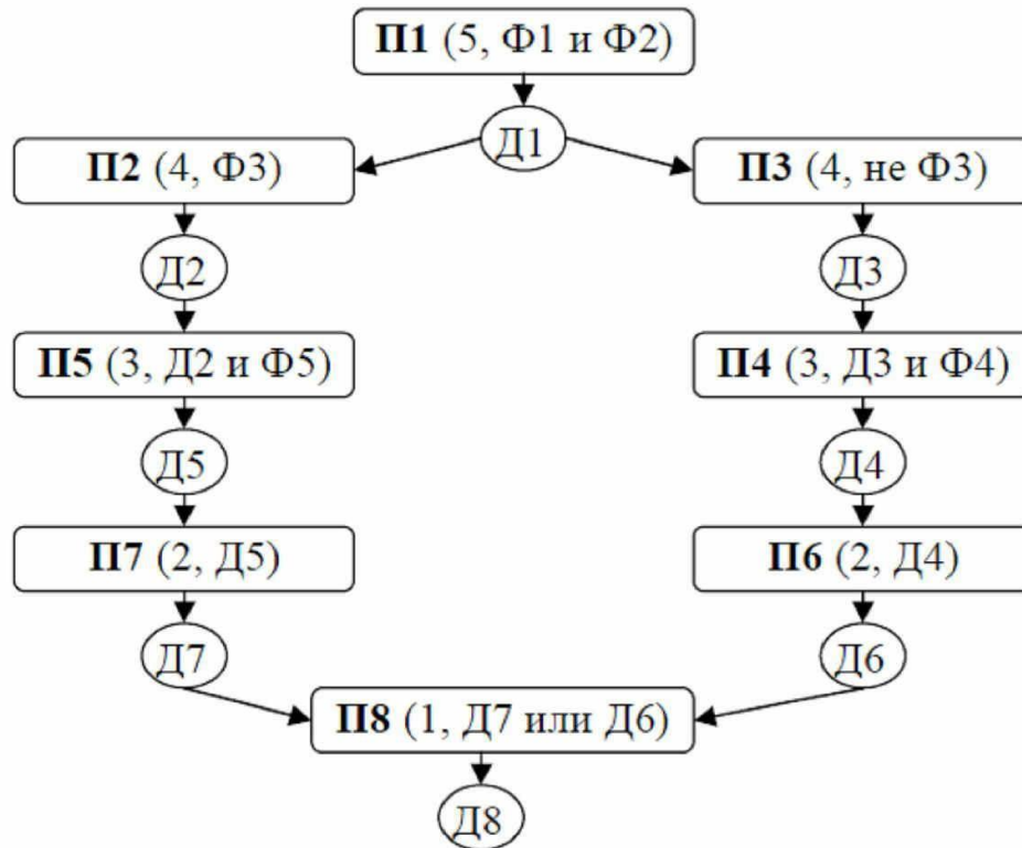
Рис. 1 – Пример графа модели знаний
