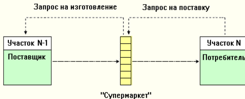
Рисунок 1.2 - Схема восполнения запасов «Супермаркета»
