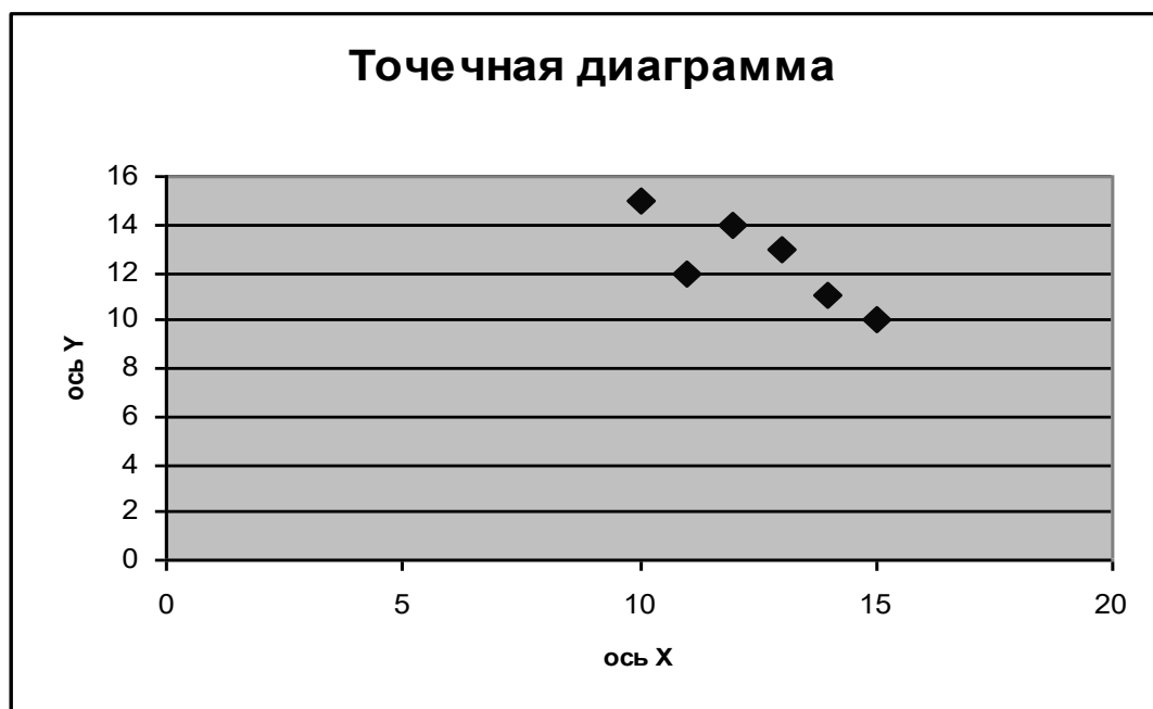
Рисунок 12 – Точечная диаграмма
