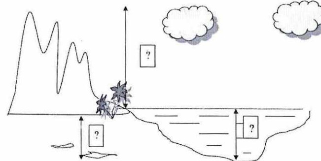
Рисунок 1. Границы биосферы
