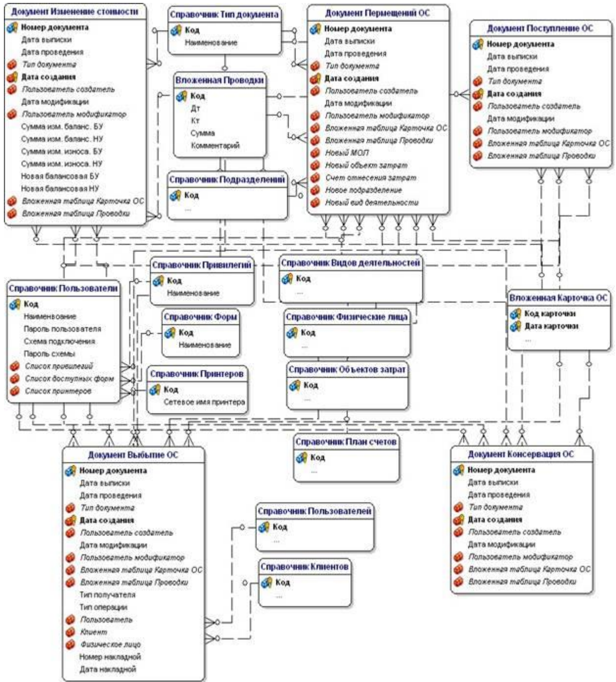
Рисунок – Инфологическая модель документов учета основных средств
