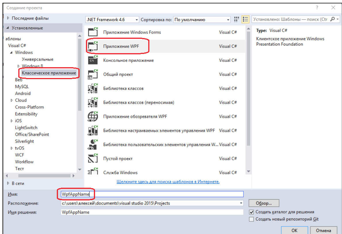
Рисунок 1.2 – создание приложения
