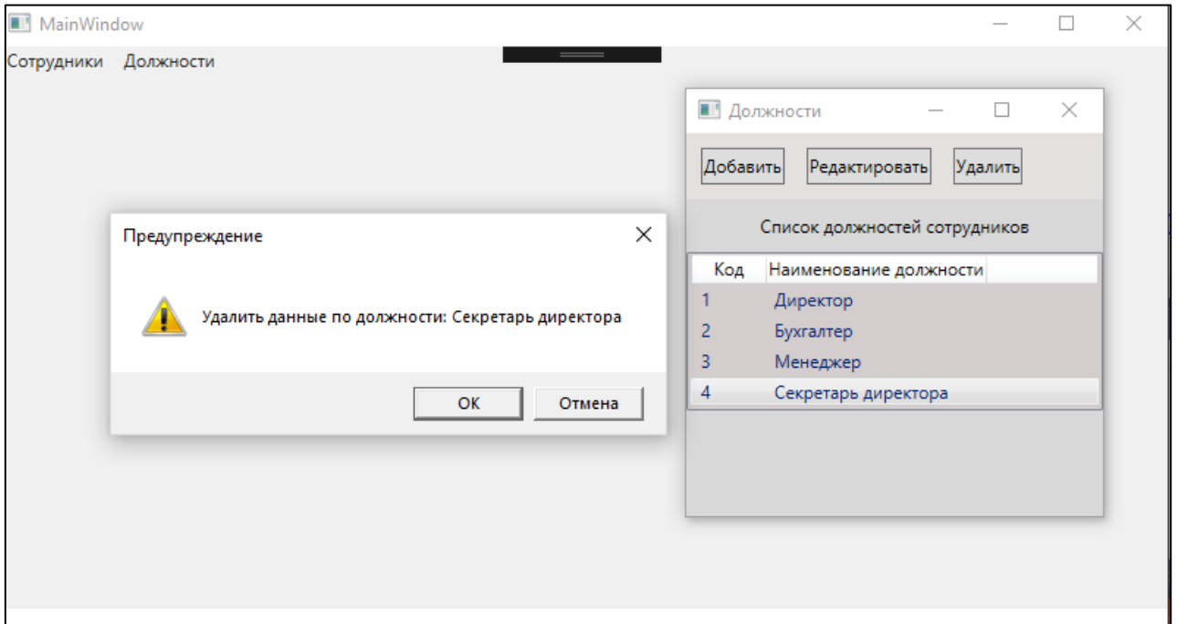
Рисунок 5.7 – Удаление должности
